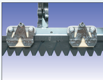
vibrationsfreier Doppelmesserbalken
